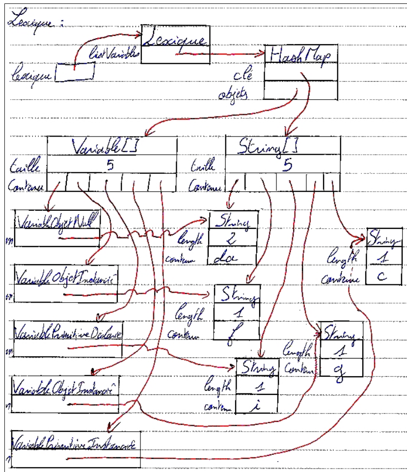
Figure 1. Représentation schématique des variables et objets en mémoire après l'exécution de quelques instructions de programme.
