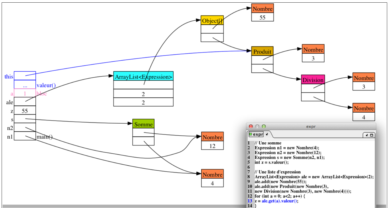
Figure 5 : Illustration du mécanisme de la liaison dynamique ; étape 2 : appel de la fonction valeur sur un objet de type dynamique Produit.
